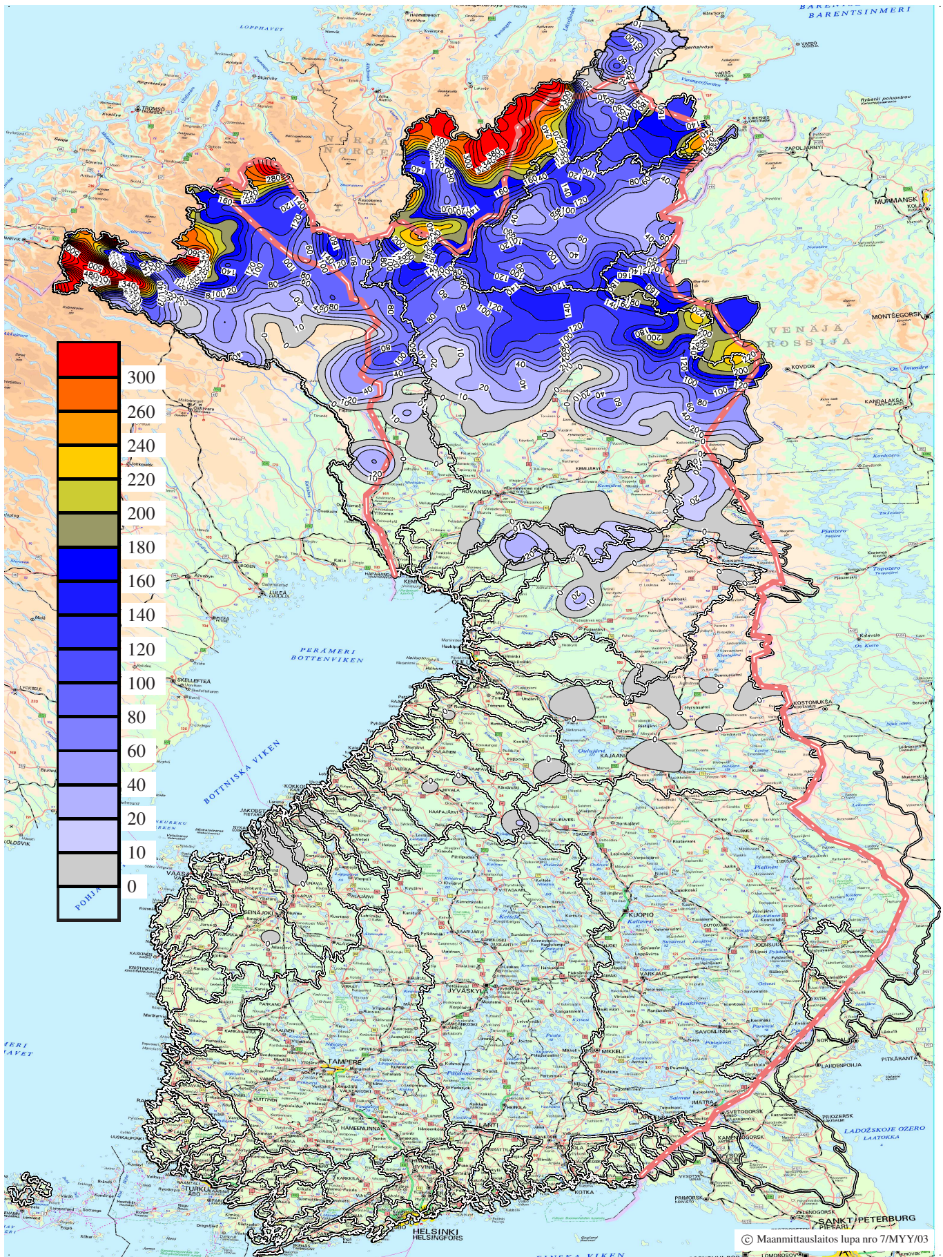
Alueen suurimmat lumikuormat (kymmenellä prosentilla alueesta lumikuorma on tätä suurempi) (kg/m 2 ) 17.5.2025 Forecast day 17. 5.
